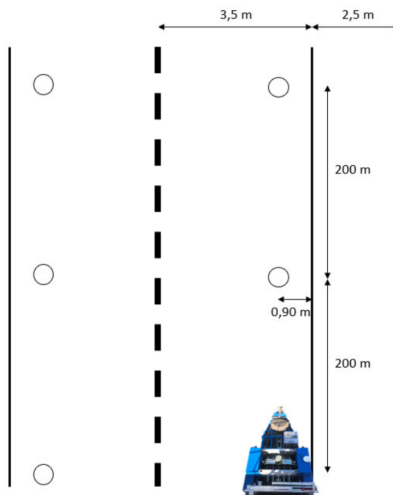
Ilustración 6 – Esquema gráfico de medición
