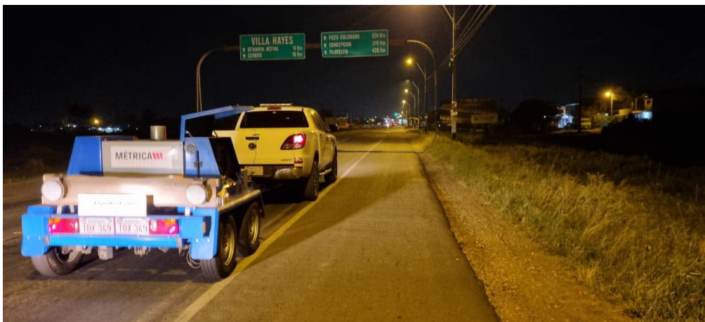
Ilustración 2 – Disposición de Equipo HWD y vehículo de tiro a 90 cm de línea de borde
