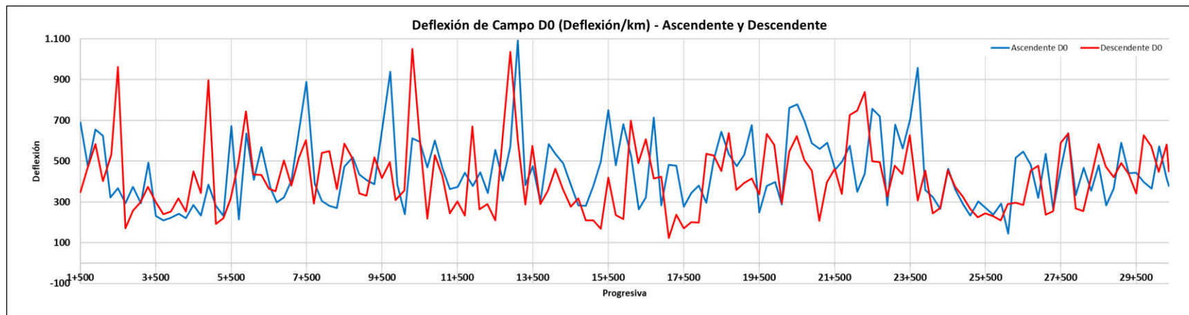
Ilustración 8 – Deflexiones D0 carril ascendente y descendente
