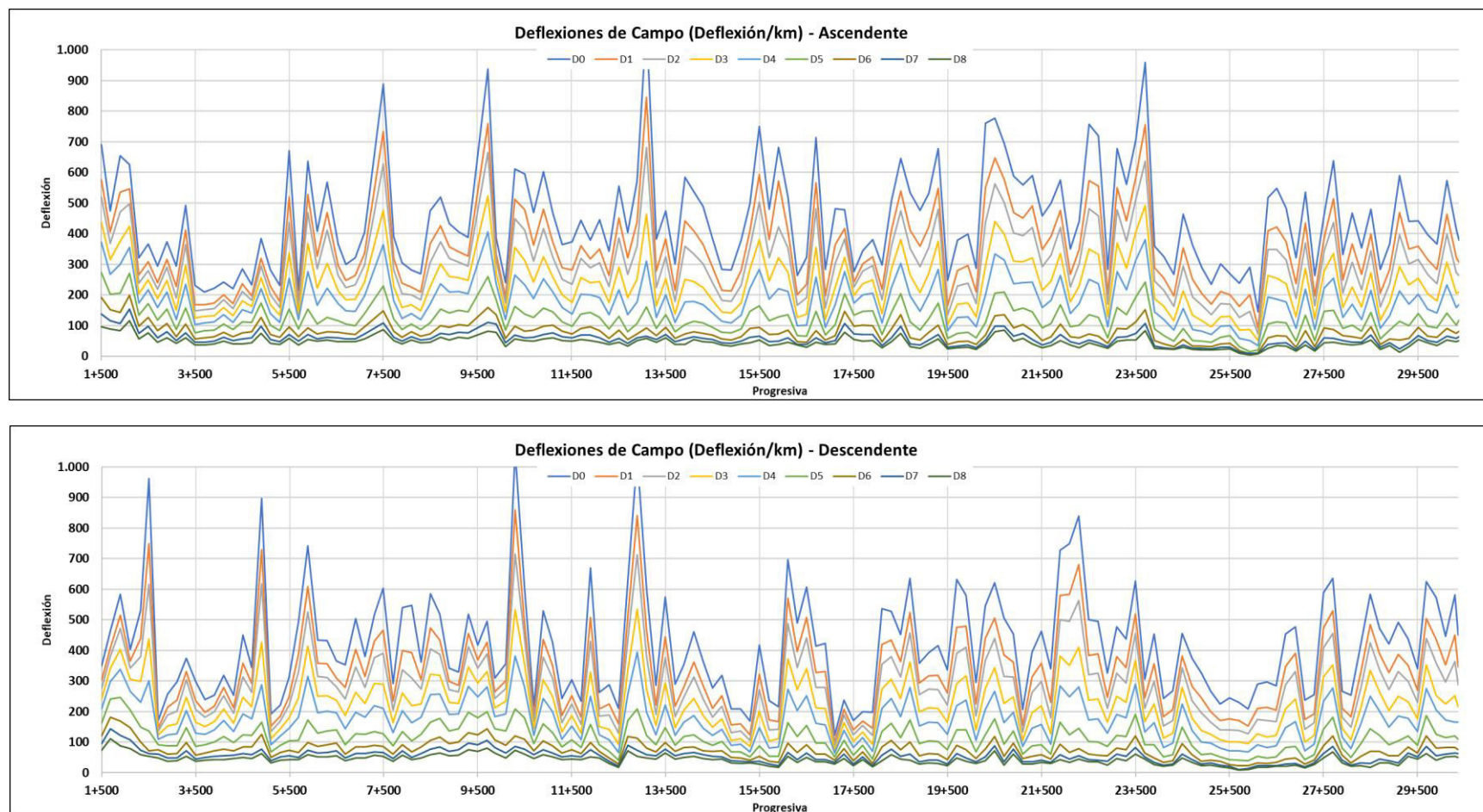
Ilustración 7 – Deflexiones por geófono ascendente y descendente
